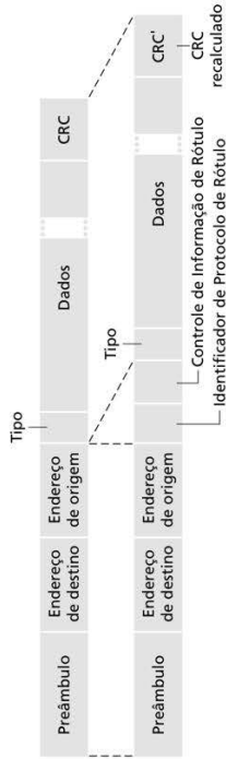
Figura 6.27 Quadro Ethernet original (no alto); quadro VLAN Ethernet 802.1Q-tagged (embaixo).
