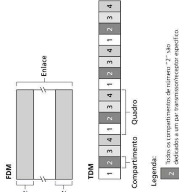
Figura 6.9 Um exemplo de TDM e FDM de quatro nós.
