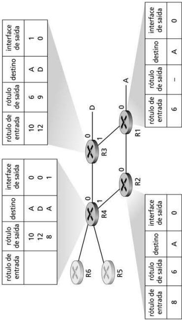
Figura 6.29 Repasse melhorado com MPLS.
